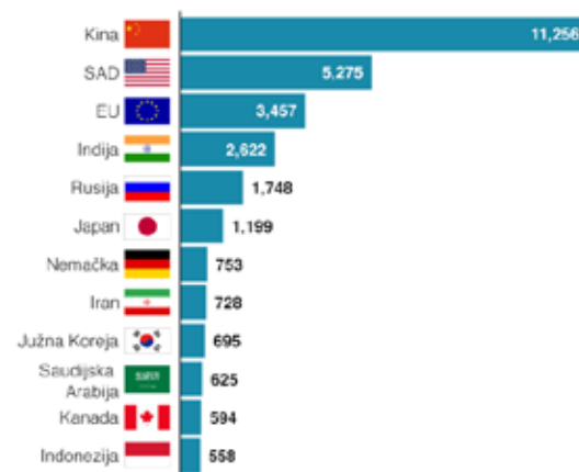
Glavni emiteri ugljen dioksida u svetu Megatona CO 2 godišnje
